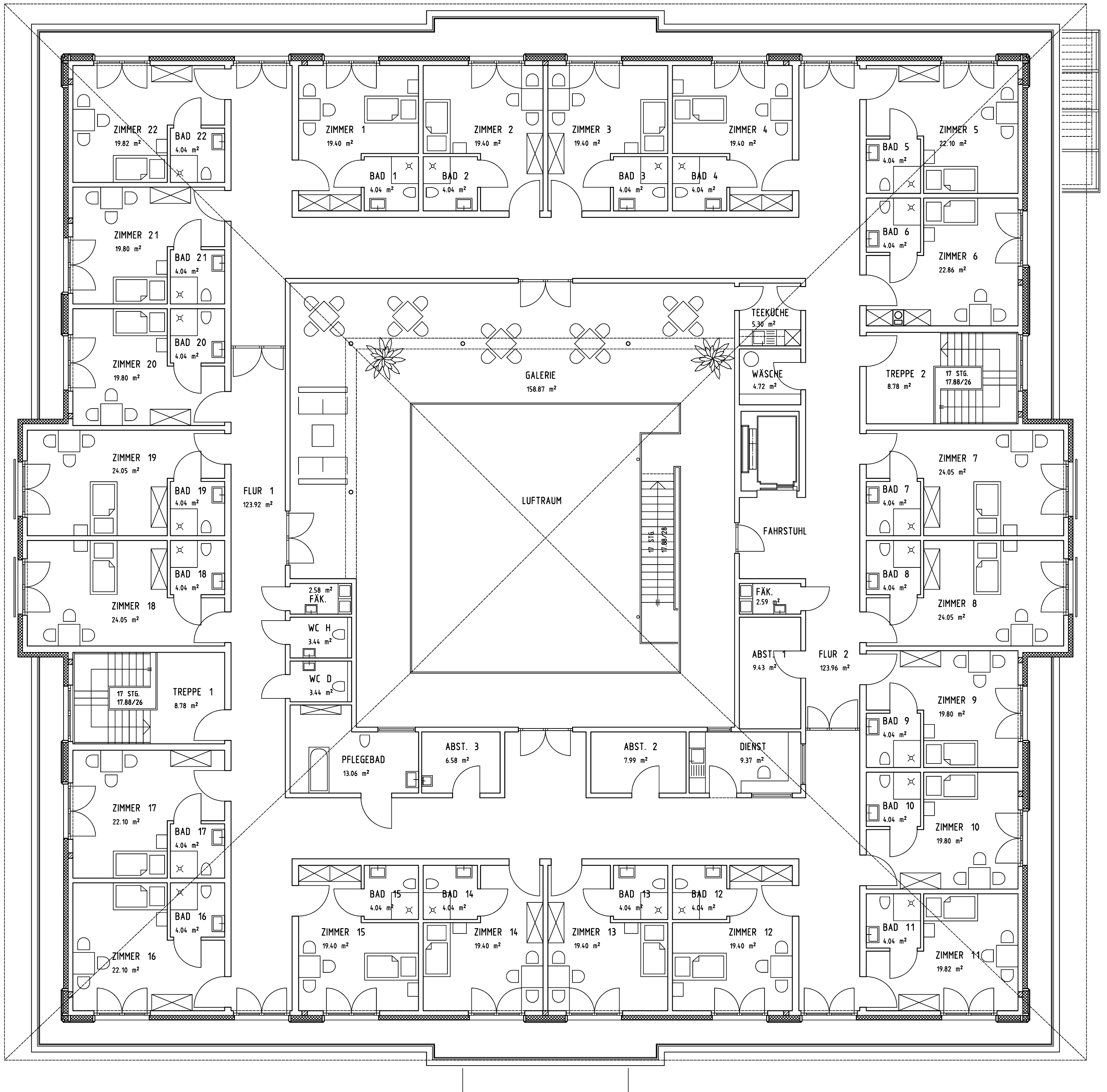
2. OBERGESCHOSS
