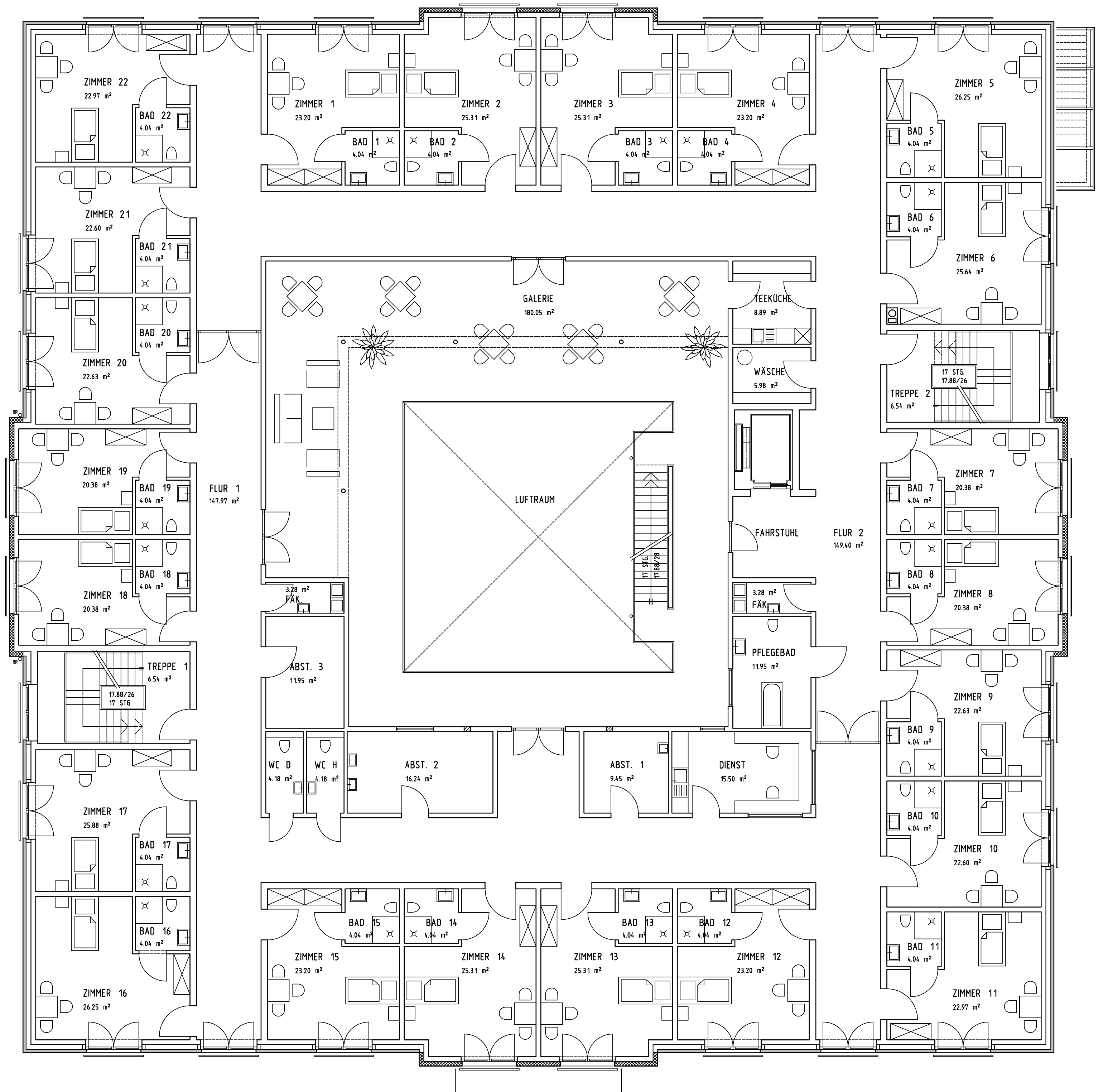
1. OBERGESCHOSS
